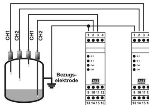
Vierkanalbetrieb mit bzw. ohne Leitungsüberwachung von CH1 durch Parallelschaltung zweier Füllstandgrenzschalter SRA – 100
