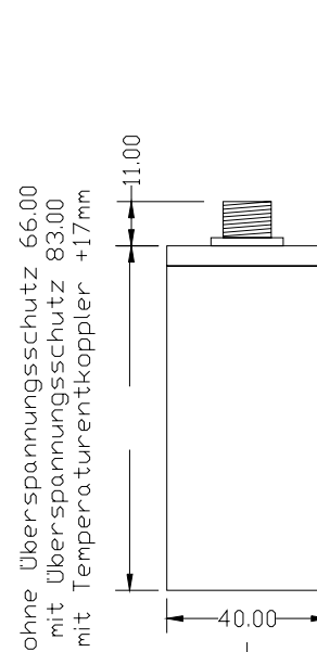
Stecker M12x1
