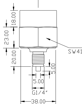
G 1/4" A nach DIN EN 837-3 TM 1
