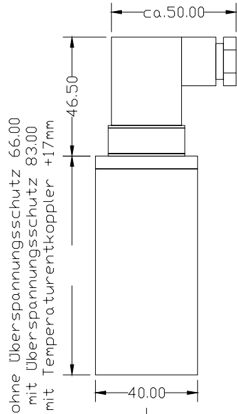
Stecker DIN EN 175-301-803-A (DIN 43650-A)
