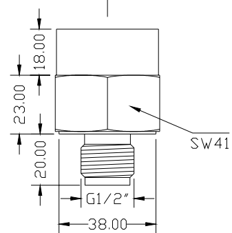
G 1/2" A mit Innenbohrung D=11,4mm TM 6
