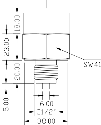
G 1/2" A nach DIN EN 837-3 TM 0
