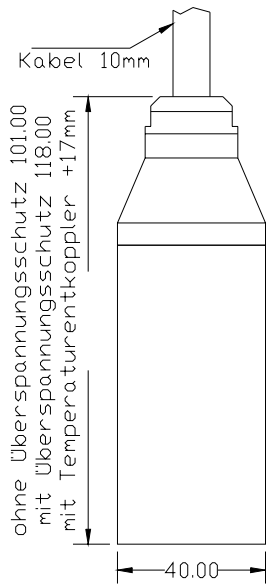
direkter Kabelabgang
