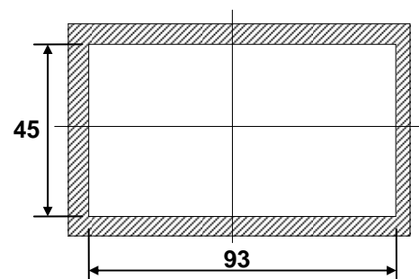
Bohrschablone
