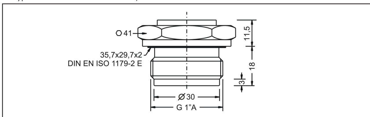
Type 5 – Thread ISO 228-1 – G1"A, front-flush
